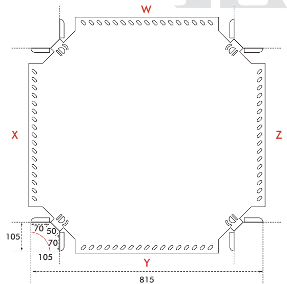
X,Y,Z,W width dimensions
